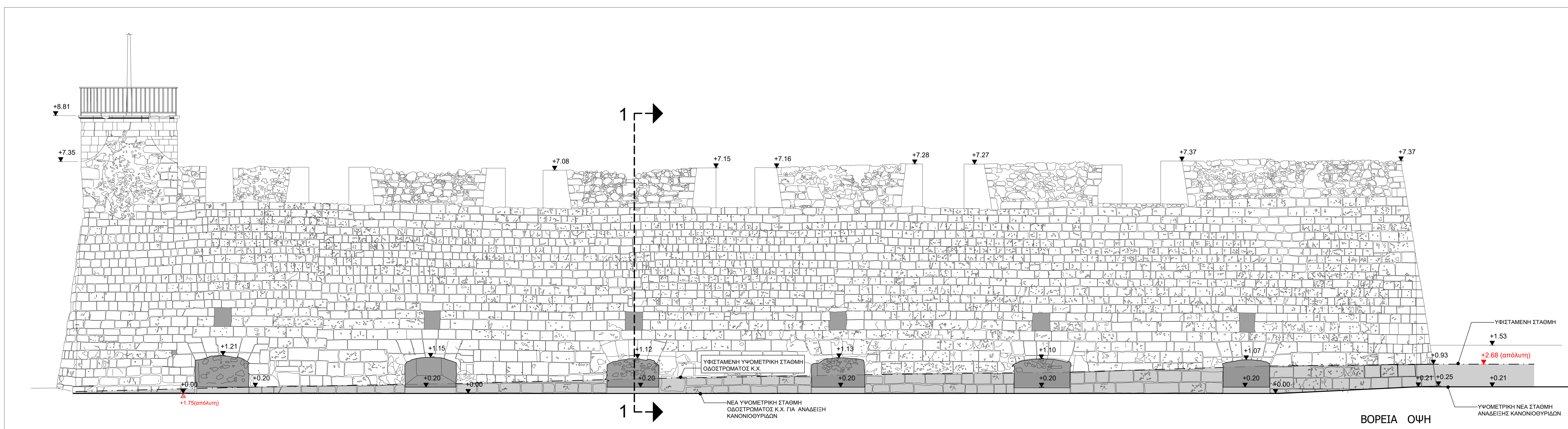
βόρεια οψη κλ. 1:50
