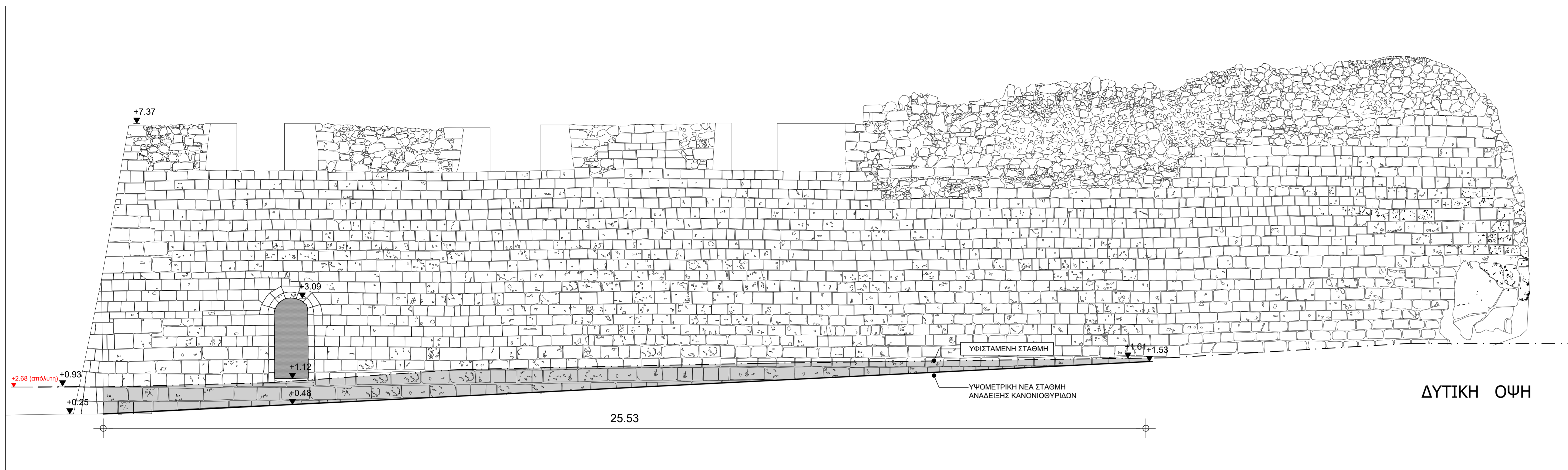
δυτική οψη κλ. 1:50
